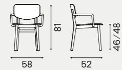
Armchair/Poltrona
