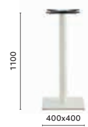
COLUMN Ø 76 TOP MAX 700x700
